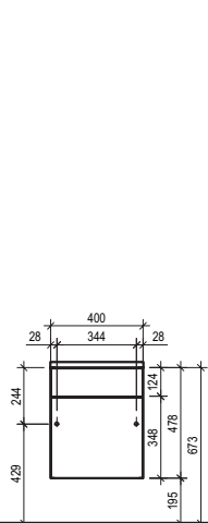
UT4F
